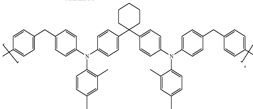
Monomer I-1
