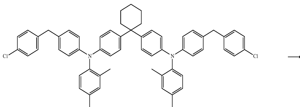
Monomer I-1
